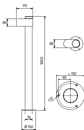
Pollare enkel för ytmontage/ Bollard single for surface mounting
