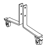
Fotvinkel med låsbara hjul l x b x h 190 x 40 x 122 mm
